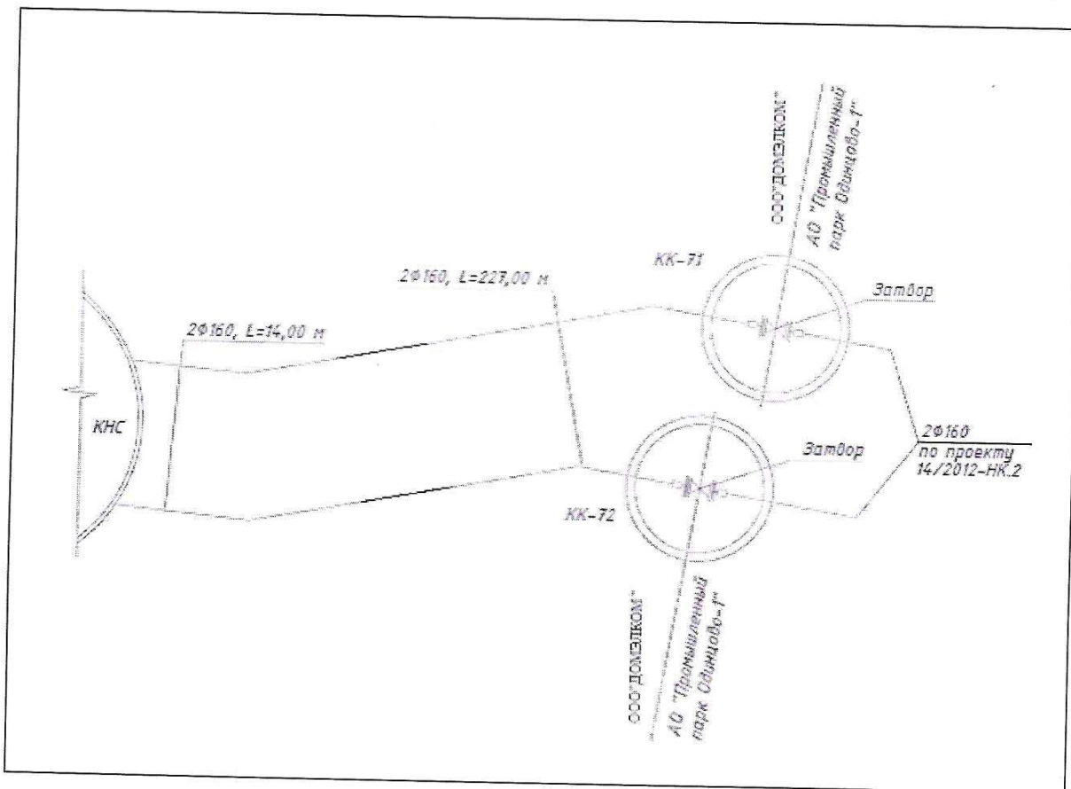
Схема границы балансовой принадлежности системы водоотведения
