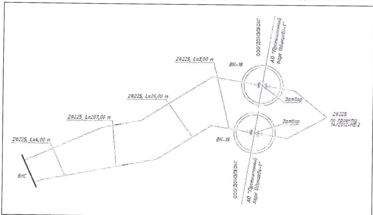
Схема границы балансовой принадлежности системы холодного водоснабжения
